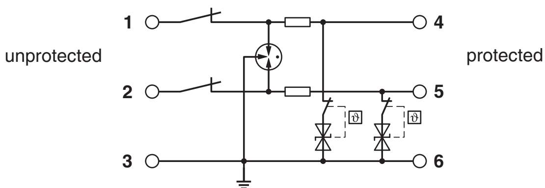
Diagrama eléctrico
