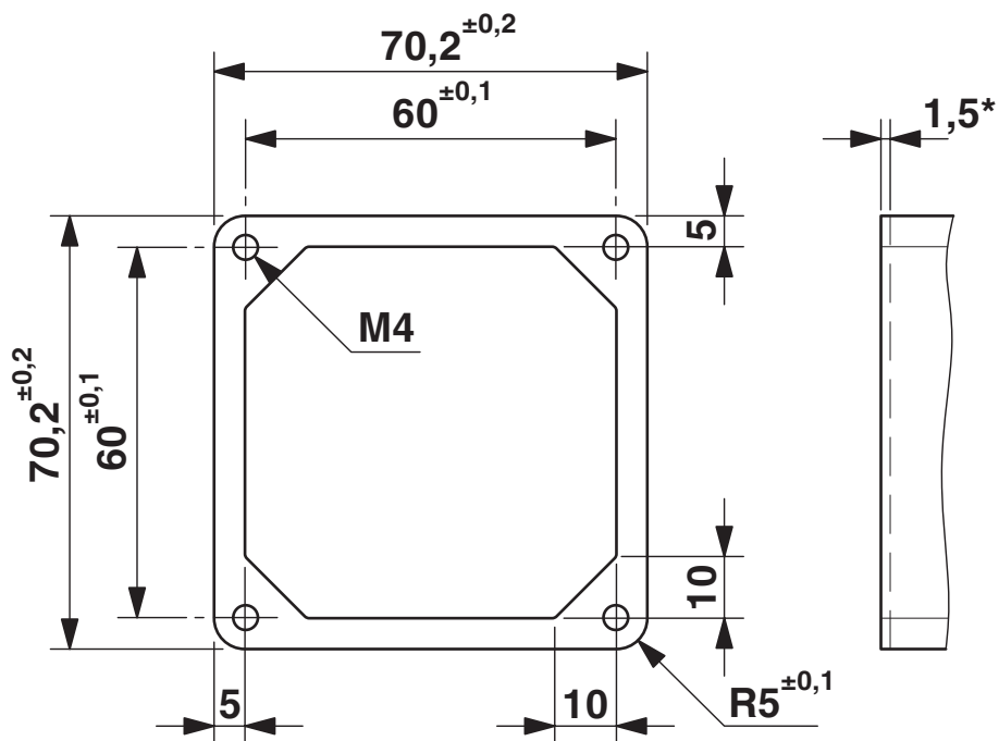
Esquema de bridas (1,5*=dimensiones interfaz mín. hasta esta altura).
