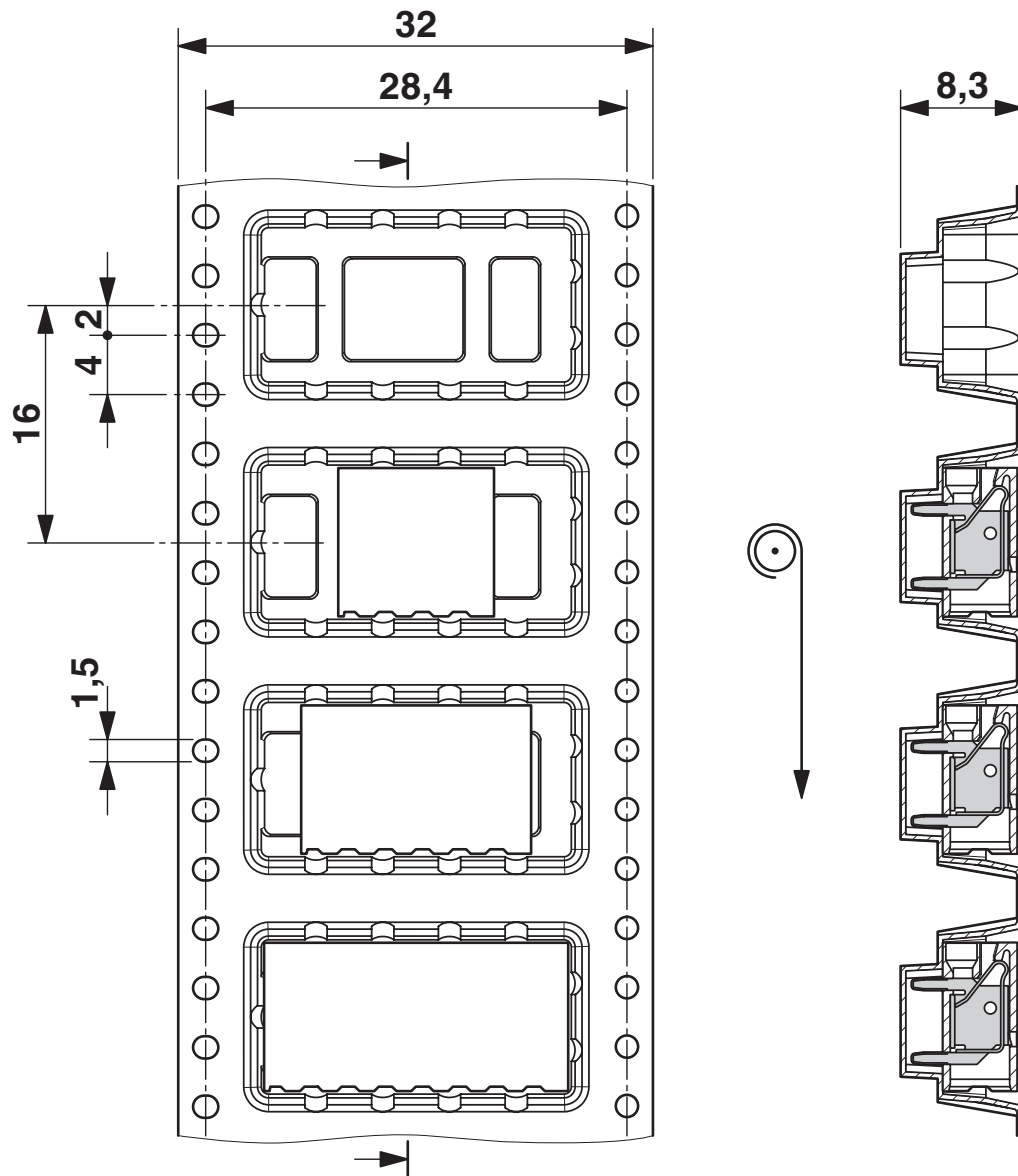
Maßzeichnung
