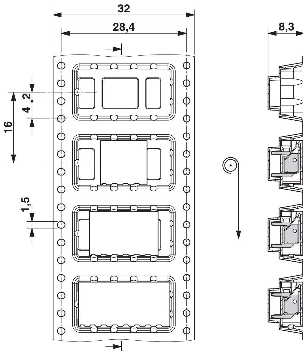
Dessin coté
