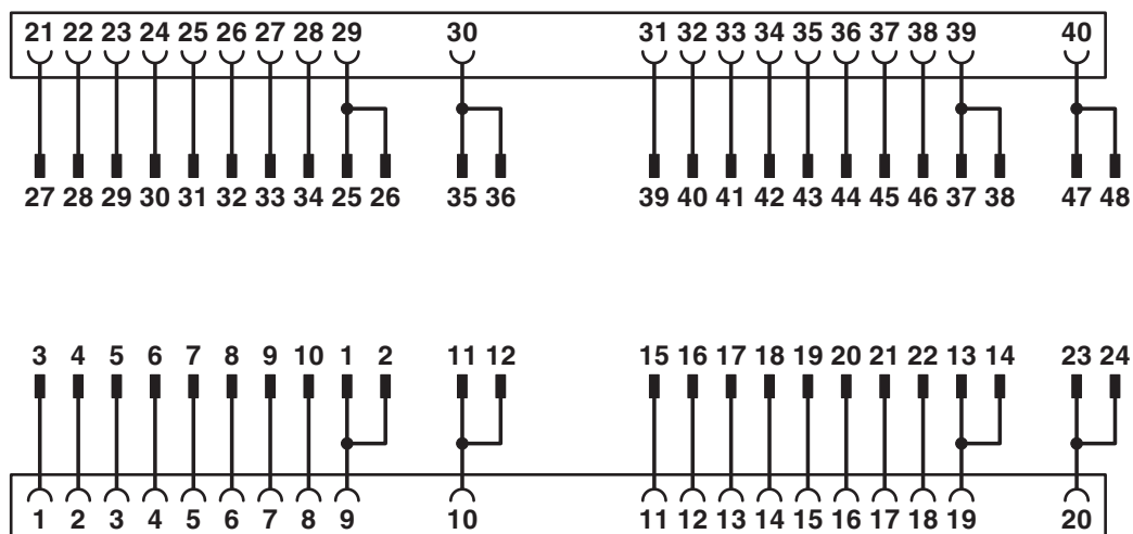
Esquema de conexiones FLKM 50-PA/AN/S7-1500
