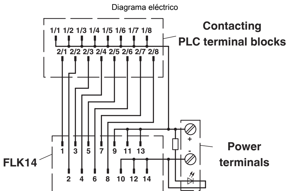
Esquema de conexiones PLC-V8L/FLK14/OUT/M
