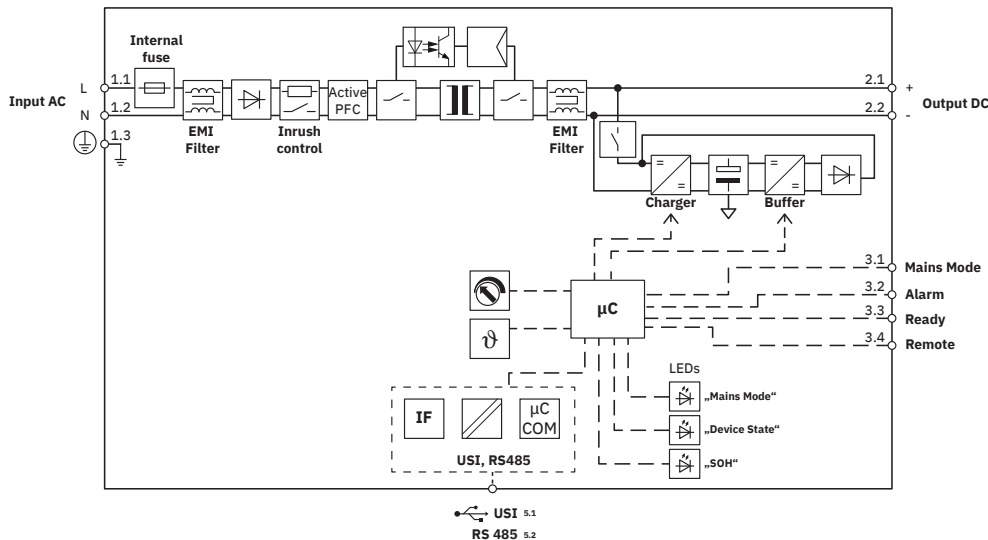
Schéma fonctionnel
