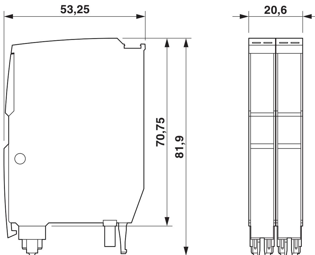
Dessin coté
