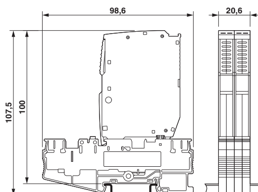
Dessin coté
