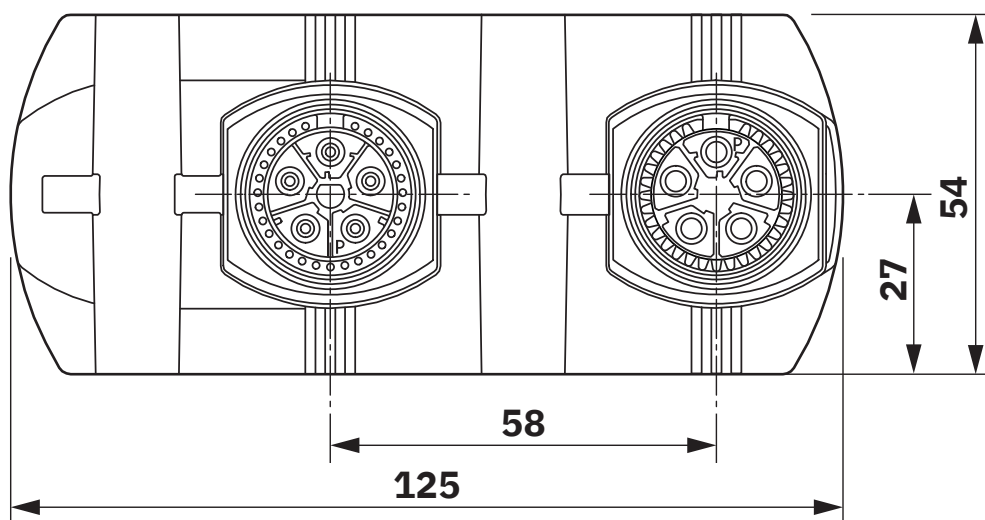
Maßzeichnung
