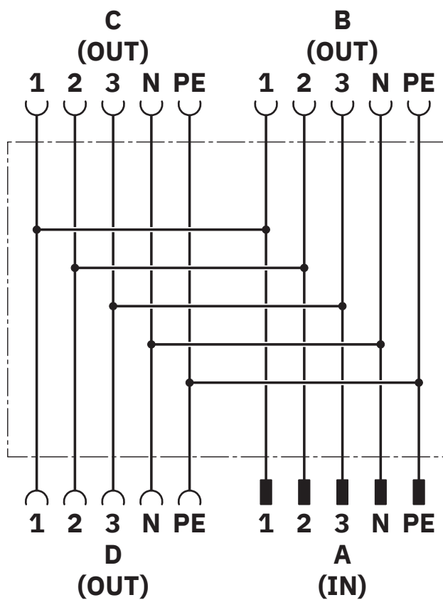
Schaltplan
