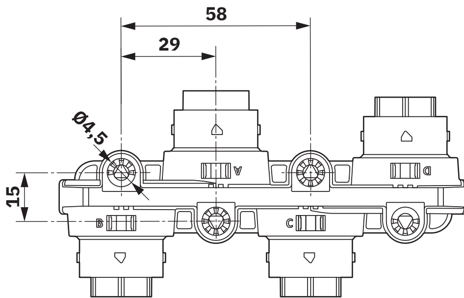
Maßzeichnung
