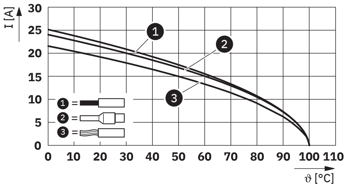
Diagrama derating para 1,5 mm 2
