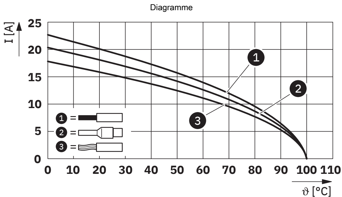
Courbe de derating pour 1,0 \text{ mm}^2
