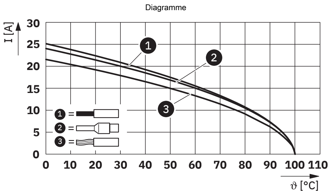
Courbe de derating pour 1,5 \text{ mm}^2
