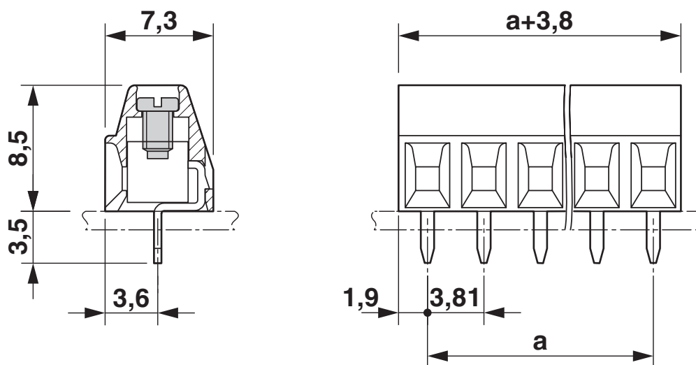
Dessin coté
