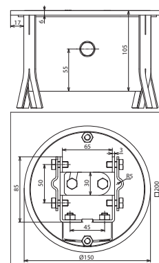
Maßbild UFTSK 7.10 FL40 200X200X105 V2A
