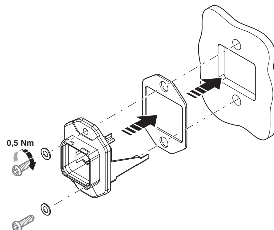
Vista desarrollada
