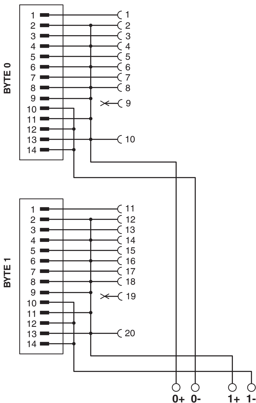
Diagrama eléctrico
