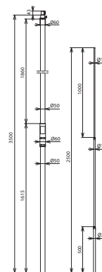
Maßbild SR D50 3500 FS22 10 2500 IP HVIP
