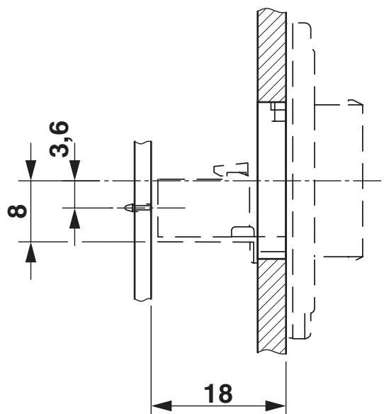
Dessin coté
