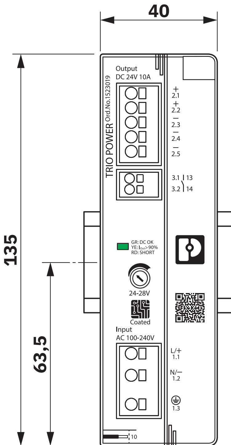
Esquema de dimensiones
