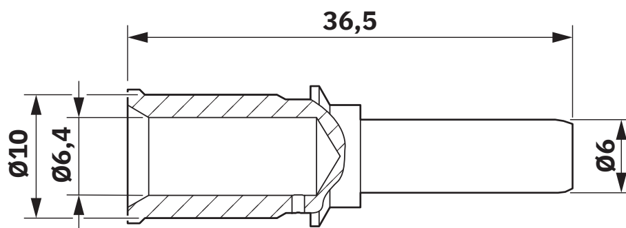
Dessin coté
