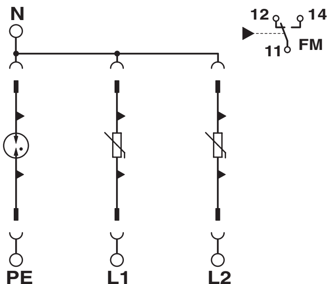
Diagrama eléctrico
