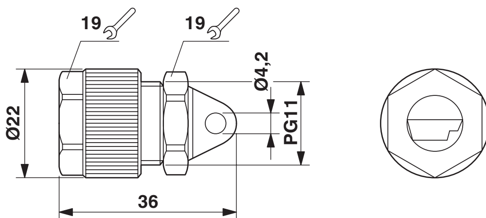
Dessin coté
