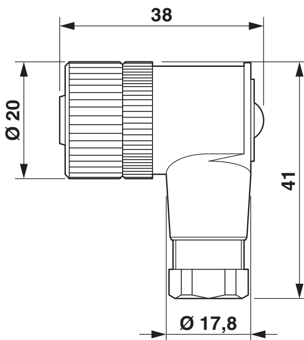
Dessin coté
