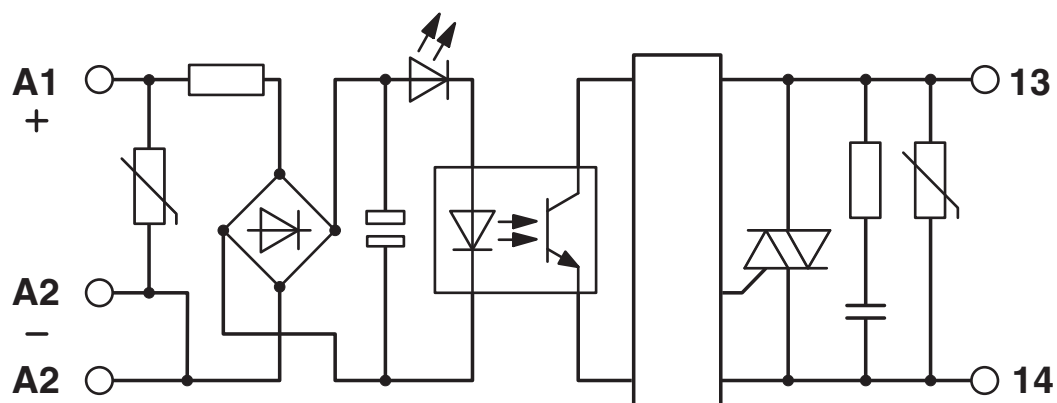
Diagrama eléctrico
