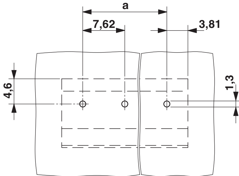
Bohrplan/Lötpadgeometrie
