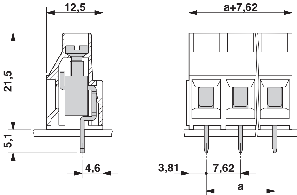
Maßzeichnung
