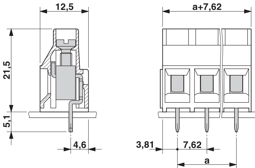
Dessin coté
