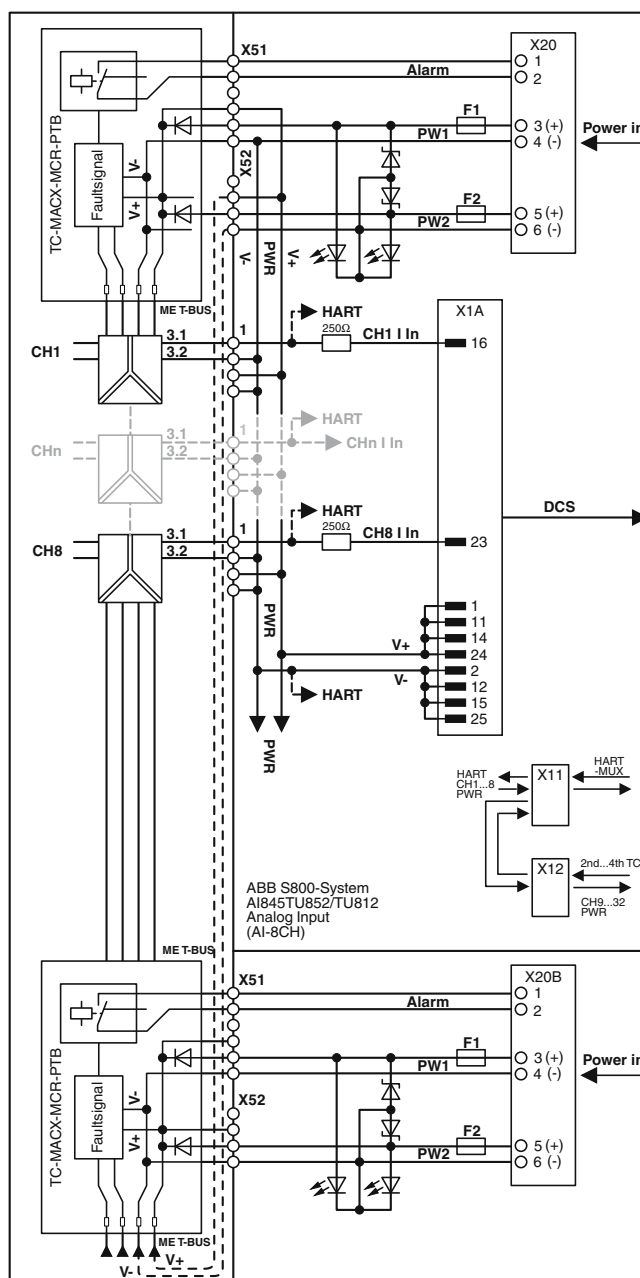
Schéma fonctionnel
