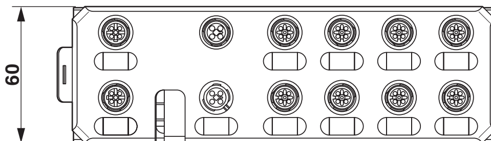
Dibujo de conexión
