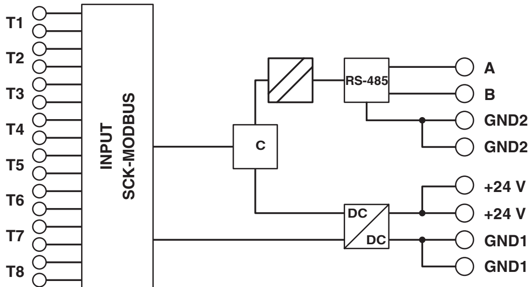
Schéma fonctionnel
