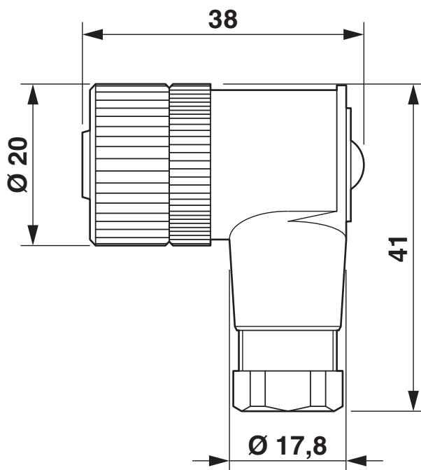
Maßzeichnung
