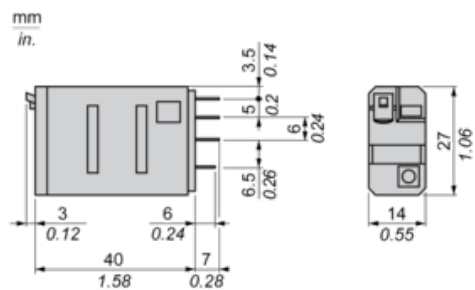
Stecker-Seitenansicht
