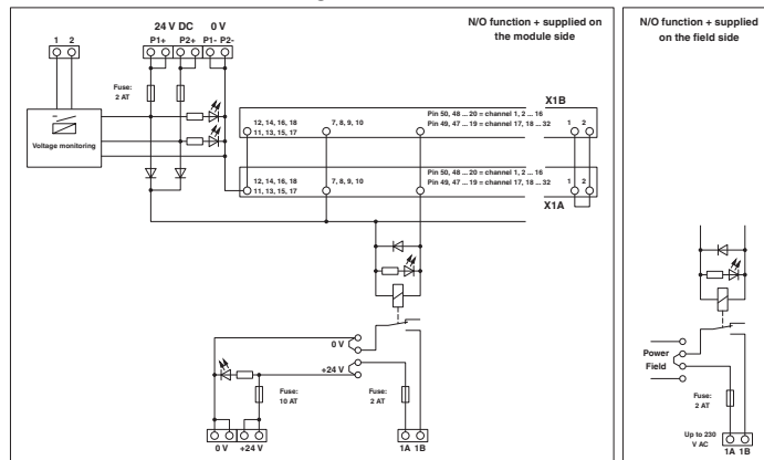
Diagrama eléctrico
