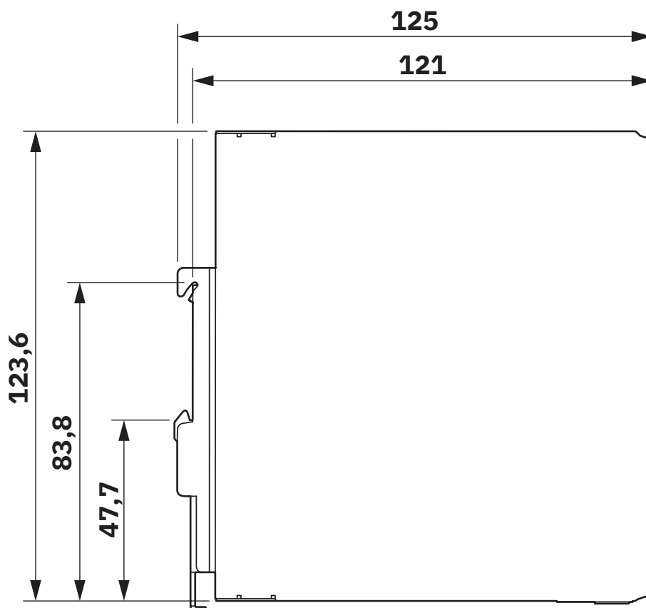
Dessin coté
