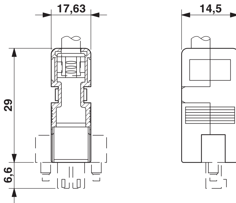
Dessin coté
