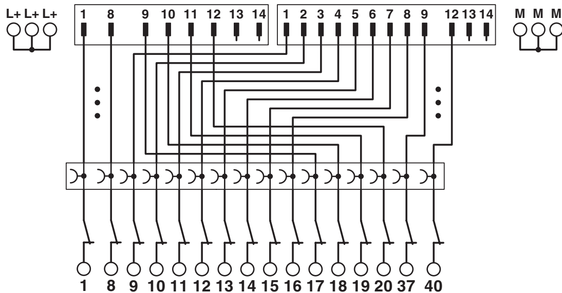
Schaltplan
