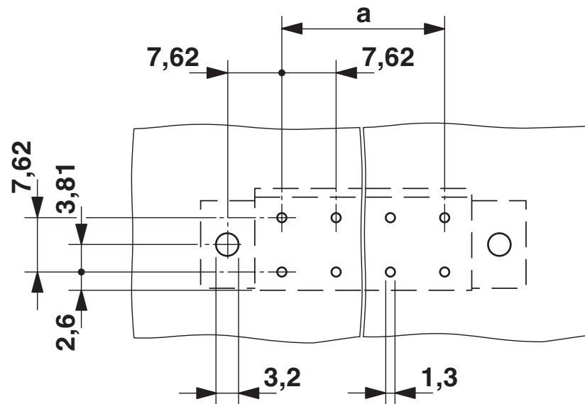
Bohrplan/Lötpadgeometrie
