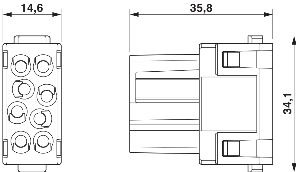
Maßzeichnung
