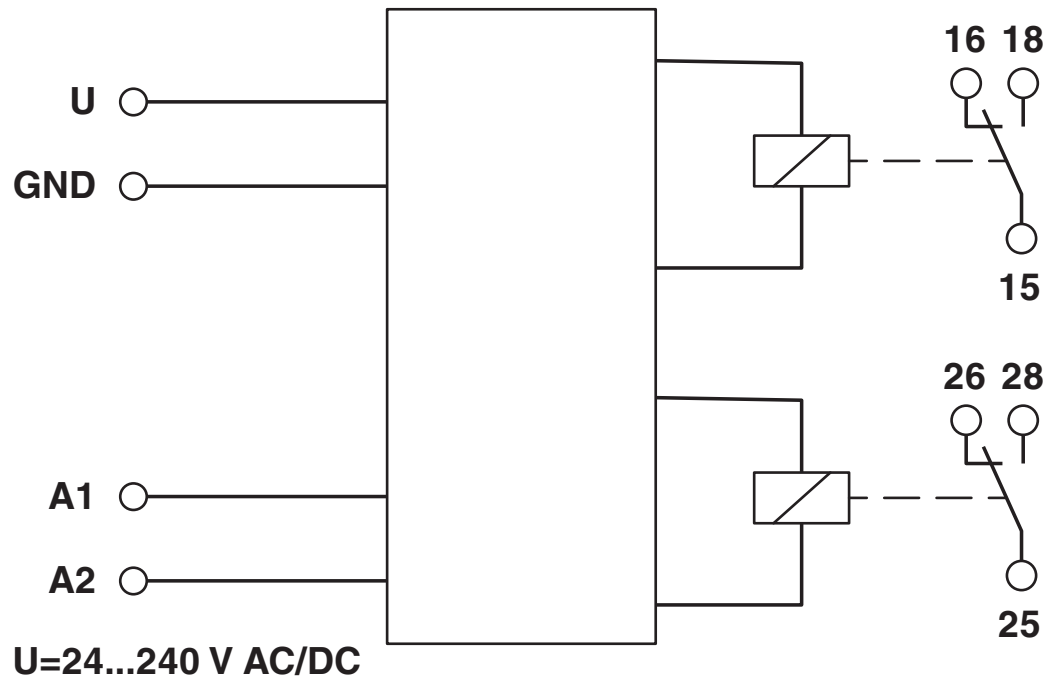
Blockschaltbild
