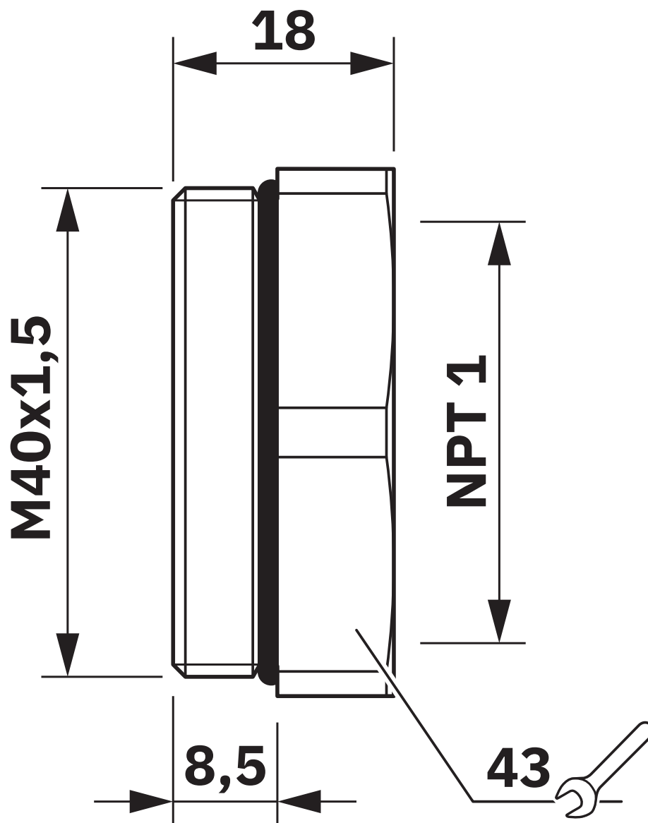
Esquema de dimensiones
