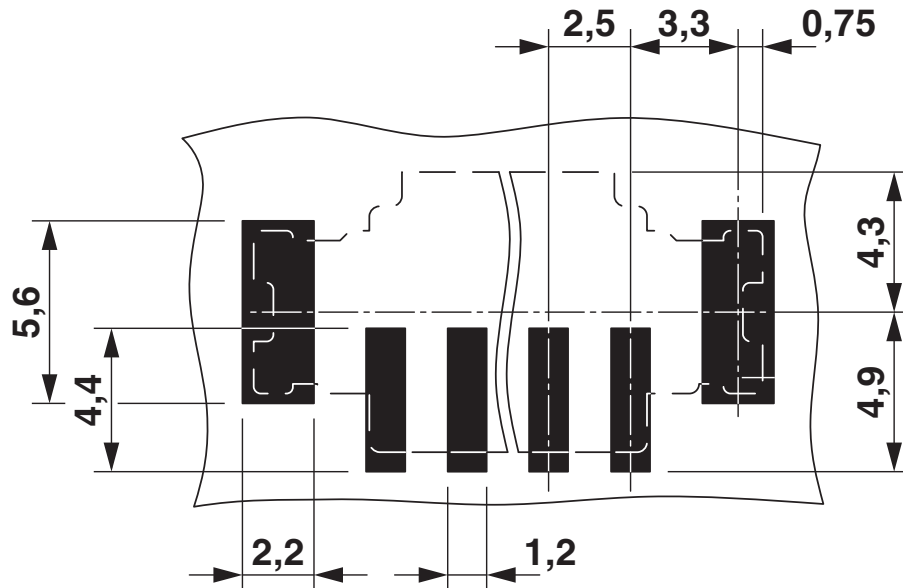
Bohrplan/Lötpadgeometrie
