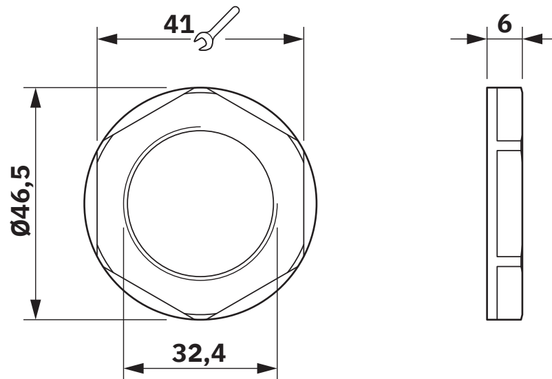
Dessin coté
