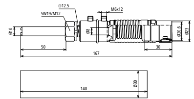
Maßbild AE ISO RAV KF HVI 75 V2A
