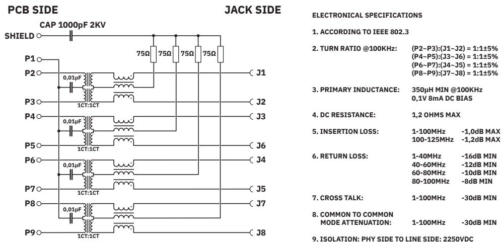
Diagrama eléctrico
