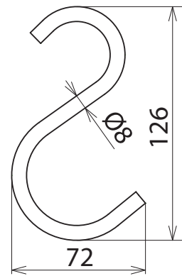
Maßbild HK 8 NS
