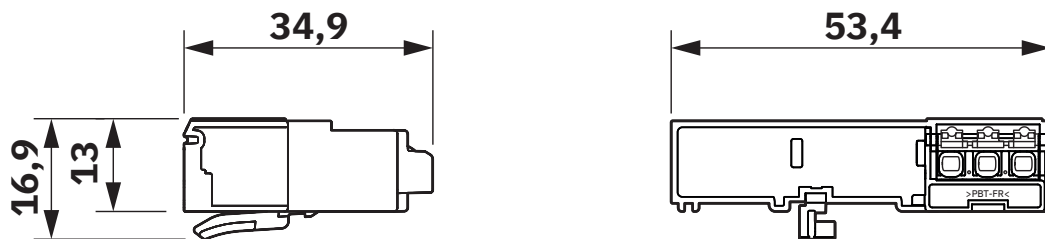
Maßzeichnung
