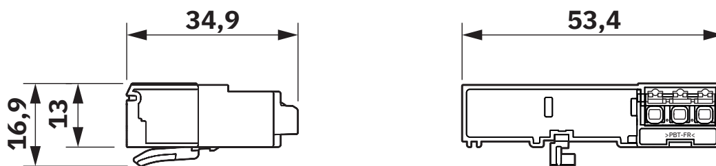
Dessin coté
