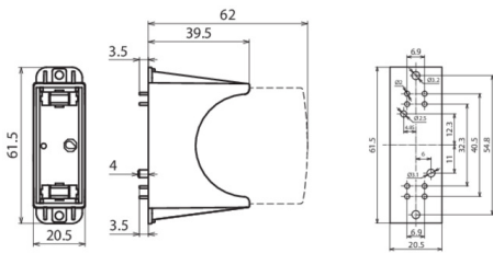
Dimensioni DG PCB PV 300
