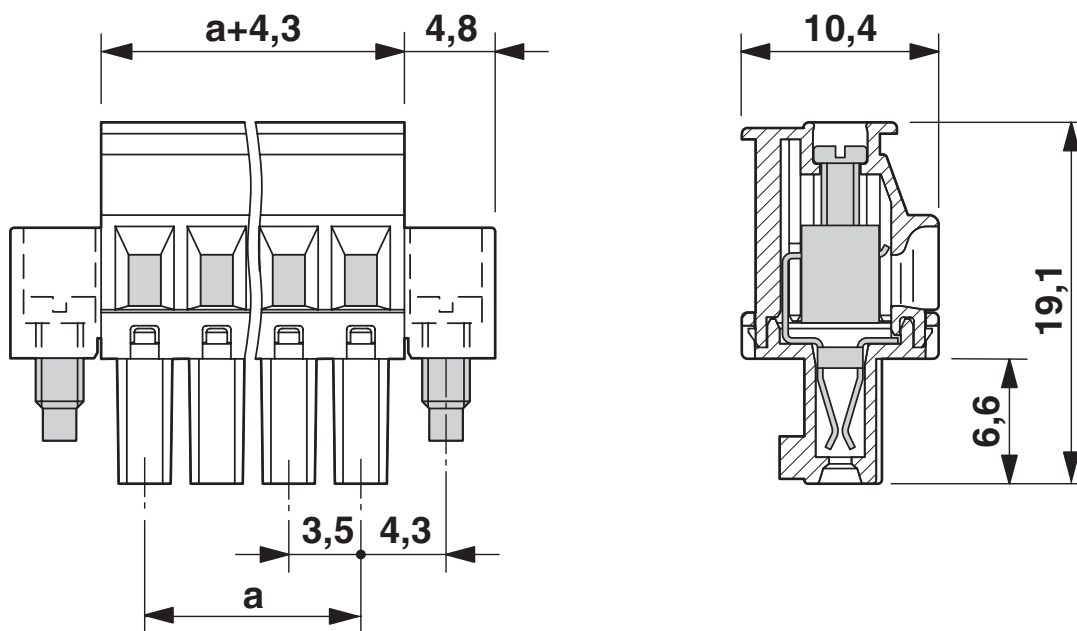
Maßzeichnung
