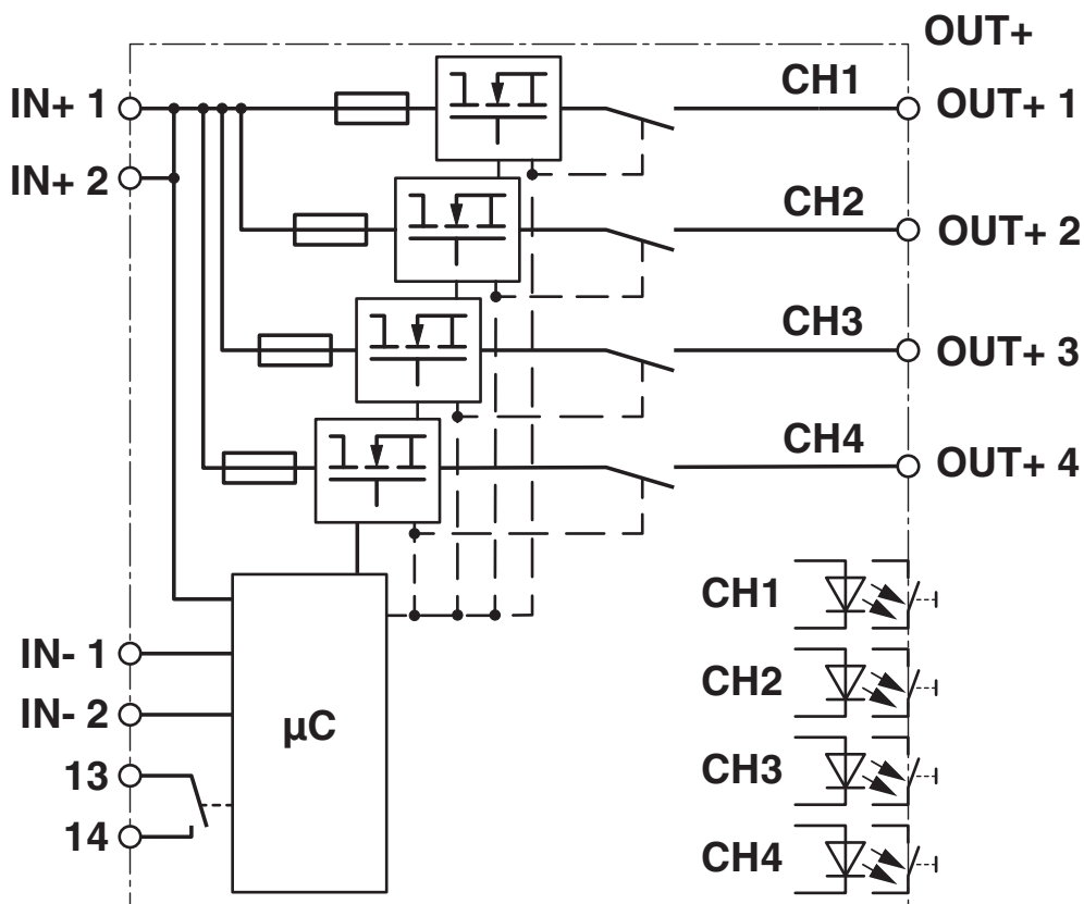
Schéma fonctionnel
