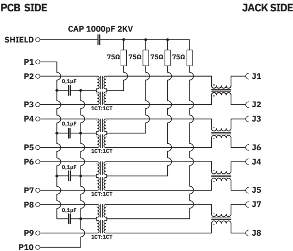
Schaltplan
