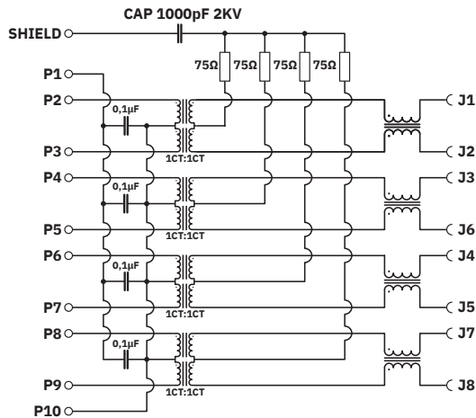
Diagrama eléctrico
